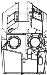
《炮塔》 Turret
